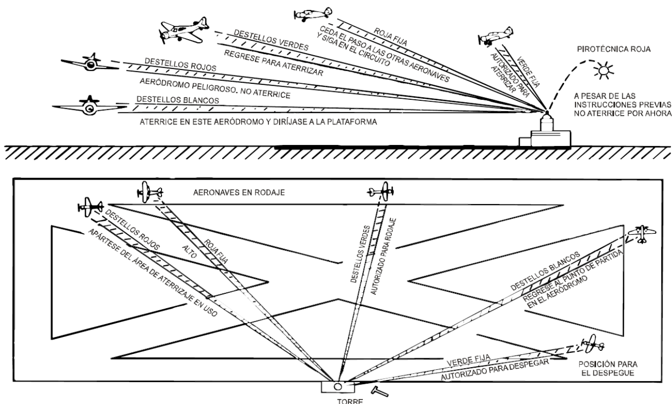
Figura 2-1.- Señales de luces para el tránsito de aeródromo.
